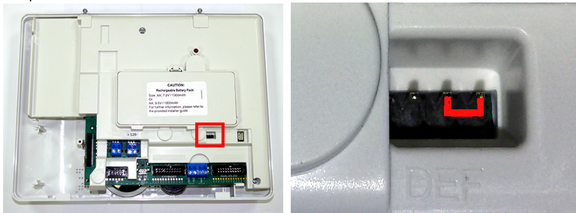
Рис.1 Панель PowerMaster-30, перемычка DEF
