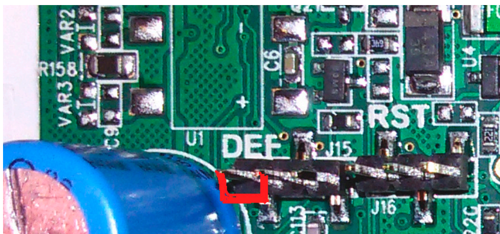
Рис.2 Панель PowerMaster-10, перемычка DEF
