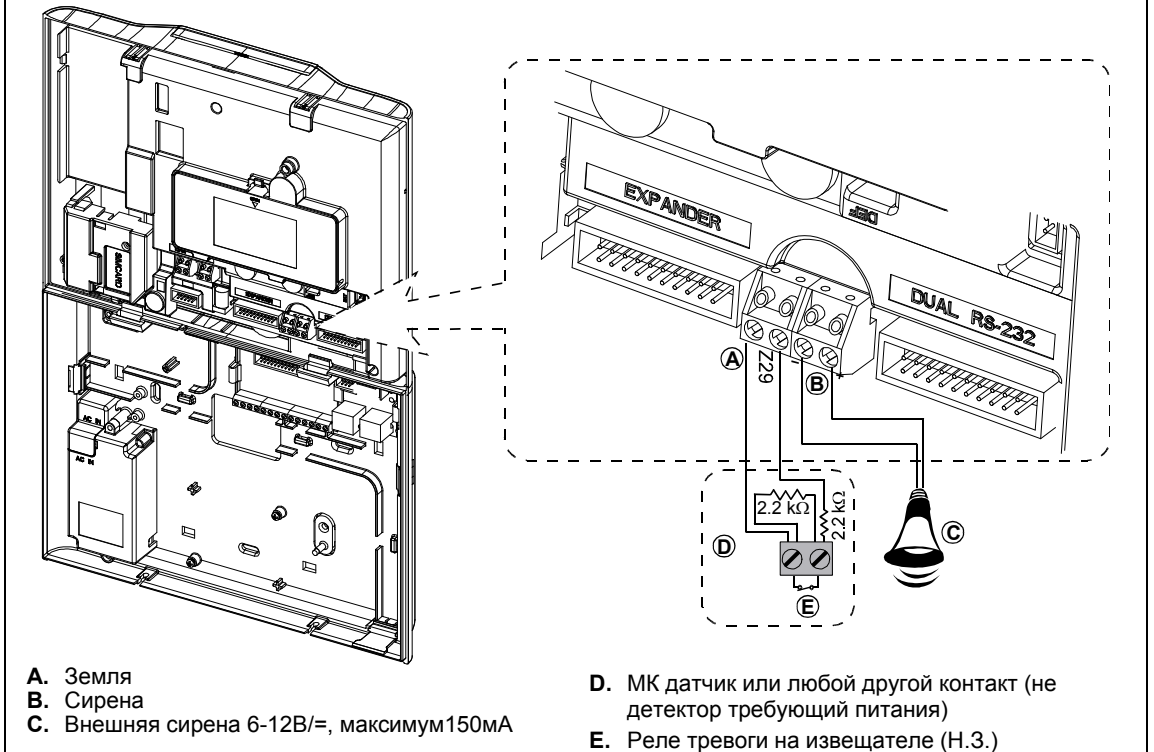
Рисунок 3.22 – Подключение зоны 29* и Сирены
