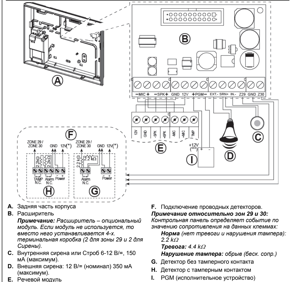
Рисунок 3.23 – Подключение устройств к модулю расширения
